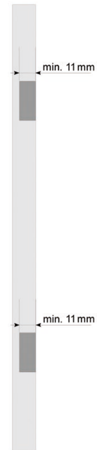
Głębokość otworów
