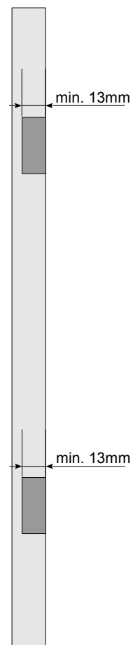
Głębokość otworów
