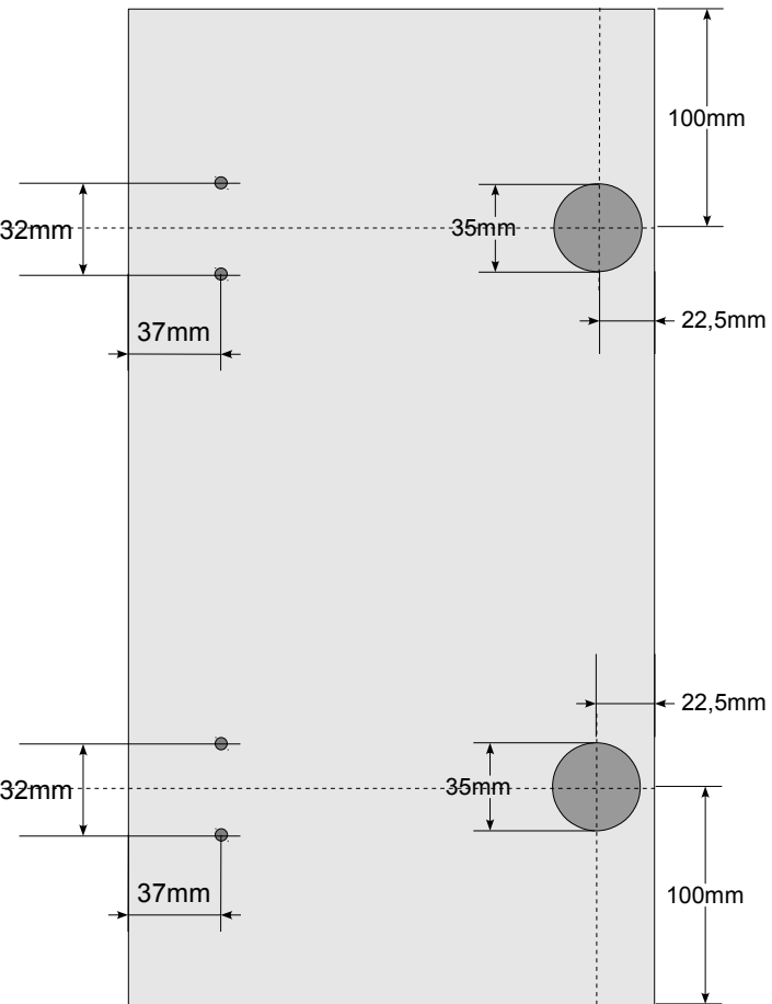
Rozmieszczenie otworów pod zawiasy na froncie
